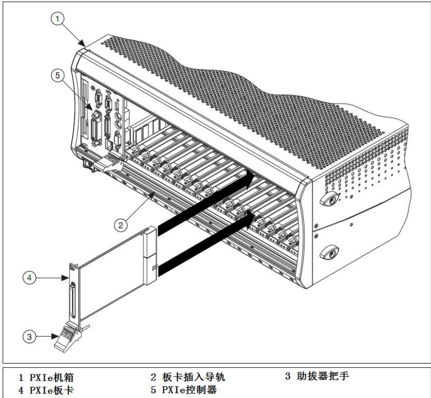
图 2-8 功能板卡插入示意图
