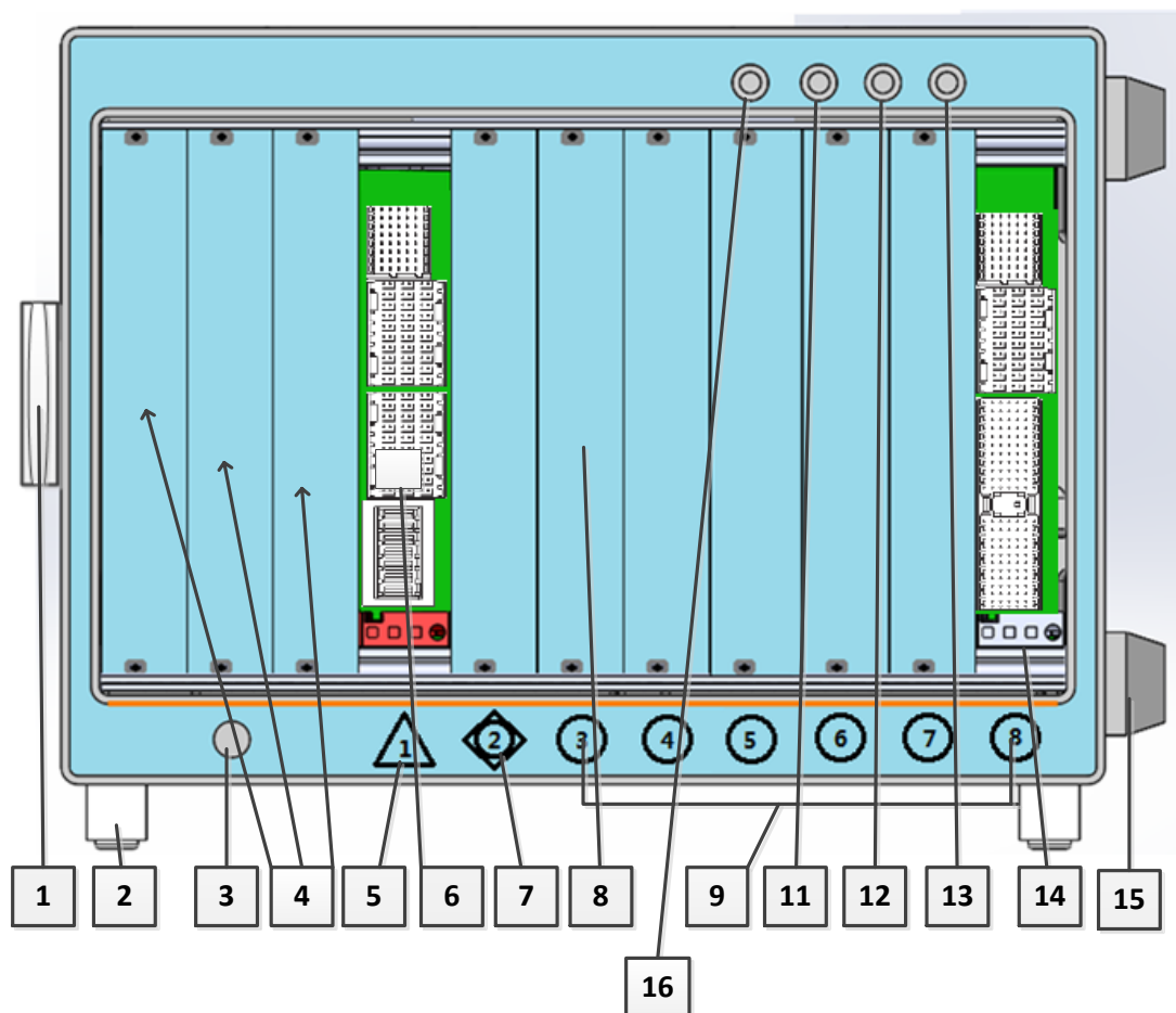
图 1-1 机箱前视图
