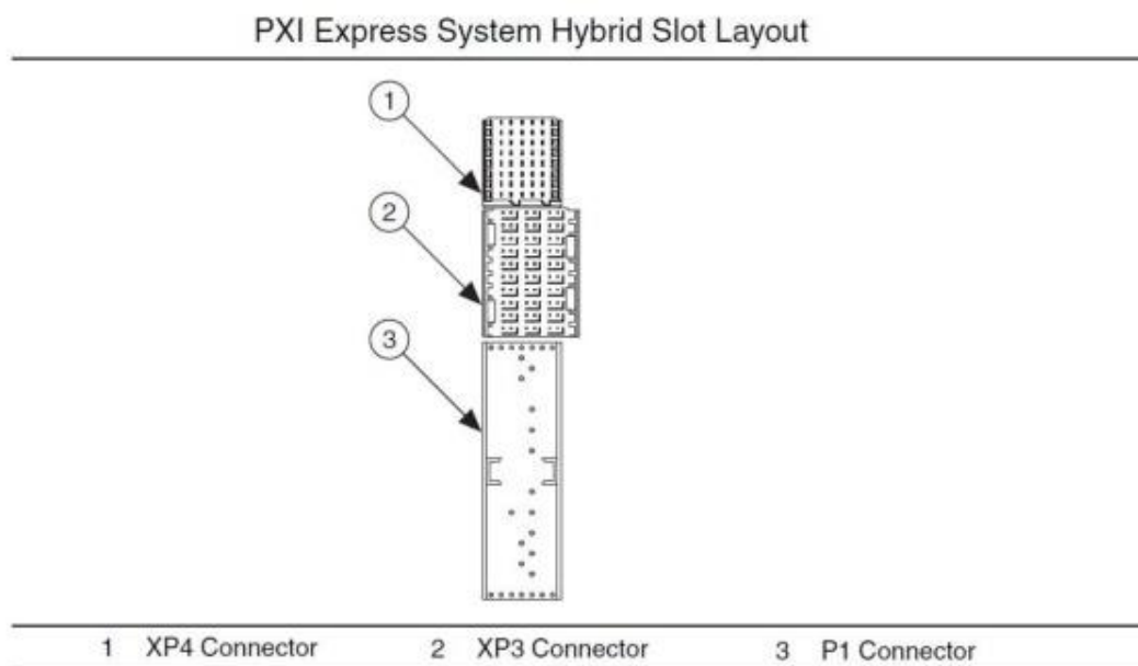
图 3-2 背板混合槽位示意图
