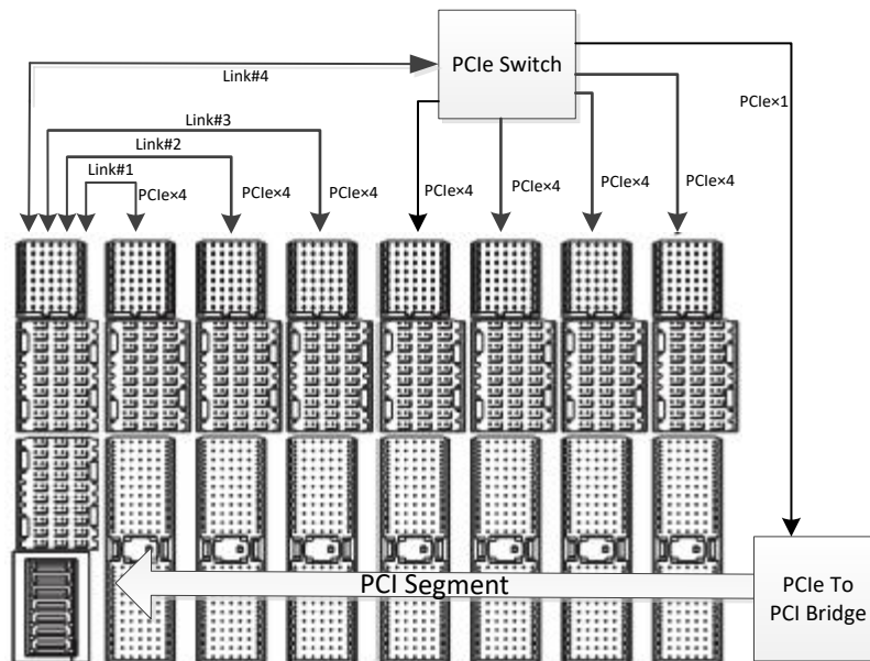
图 1-3 背板各槽位拓扑关系示意图
