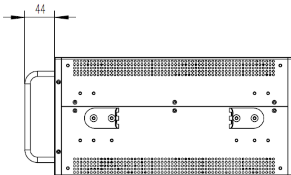
图 2-3 机箱尺寸图
