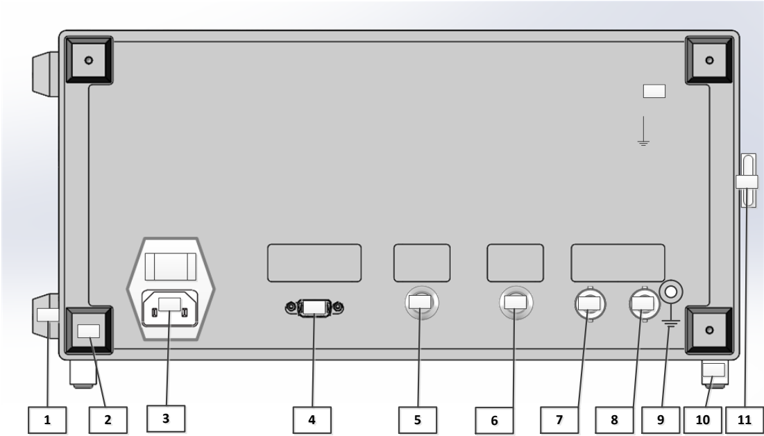
图 1-2 机箱后视图
