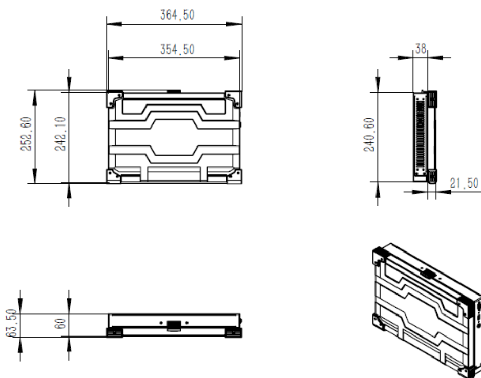
图 2-4 显示器尺寸图
