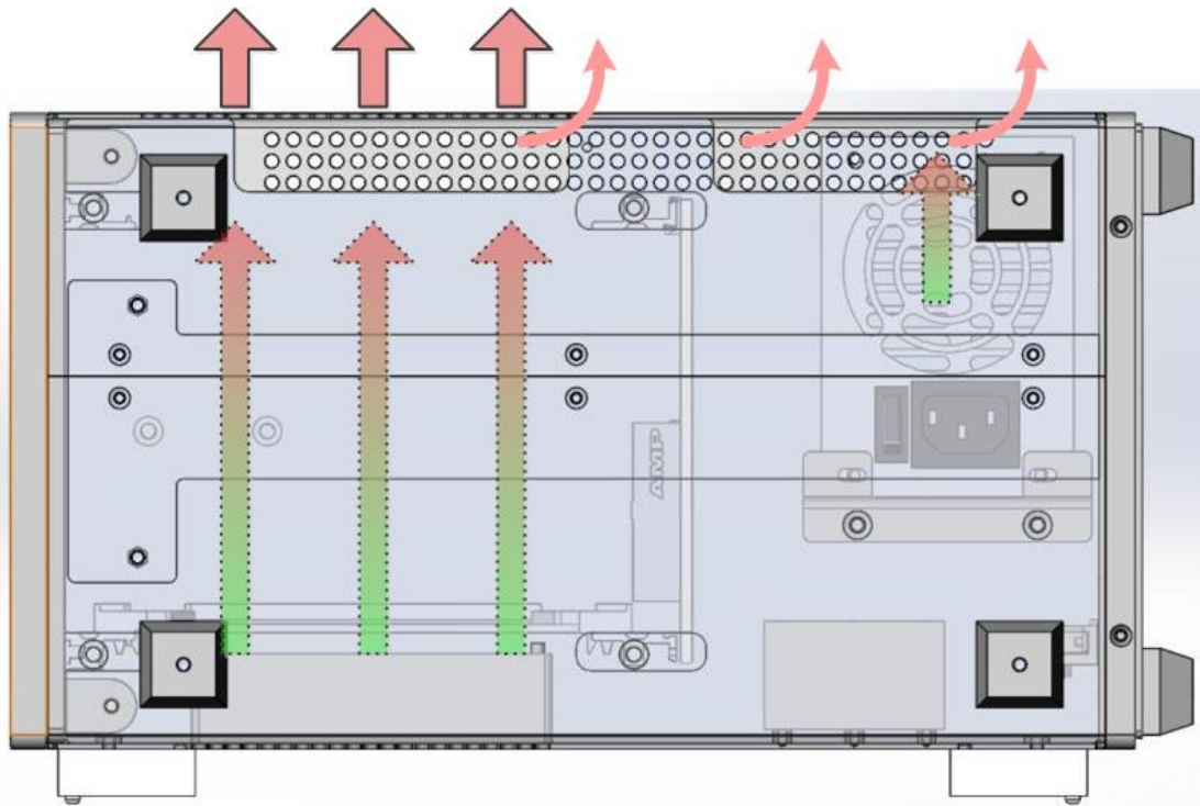
图 2-5 机箱散热通道示意图
