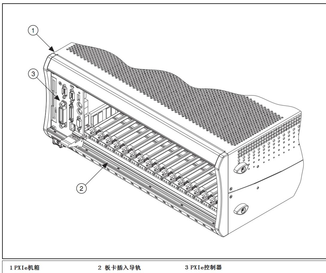
图 2-7 控制器插入机箱效果图
