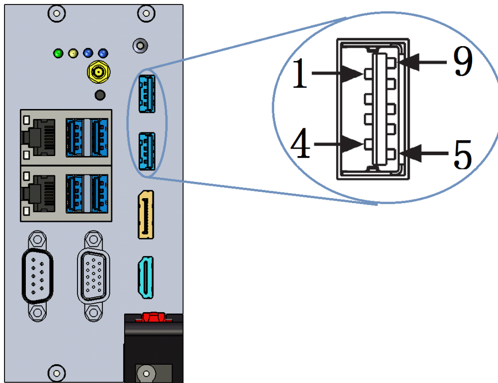
图 3-6 USB3.0 接口示意图
