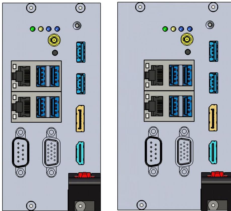
图 2-3 PXIe-3883 产品 12/16HP 面板布局图
