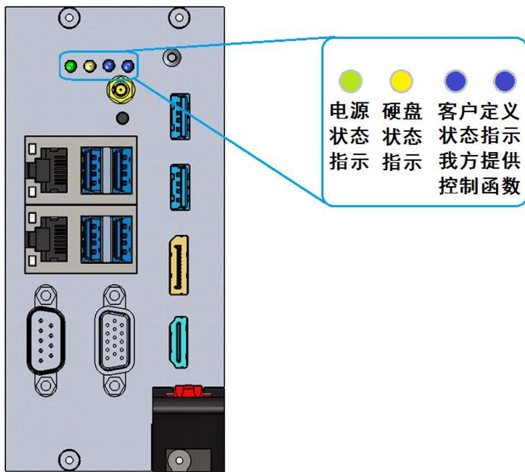
图 3-10 指示灯含义示意图
