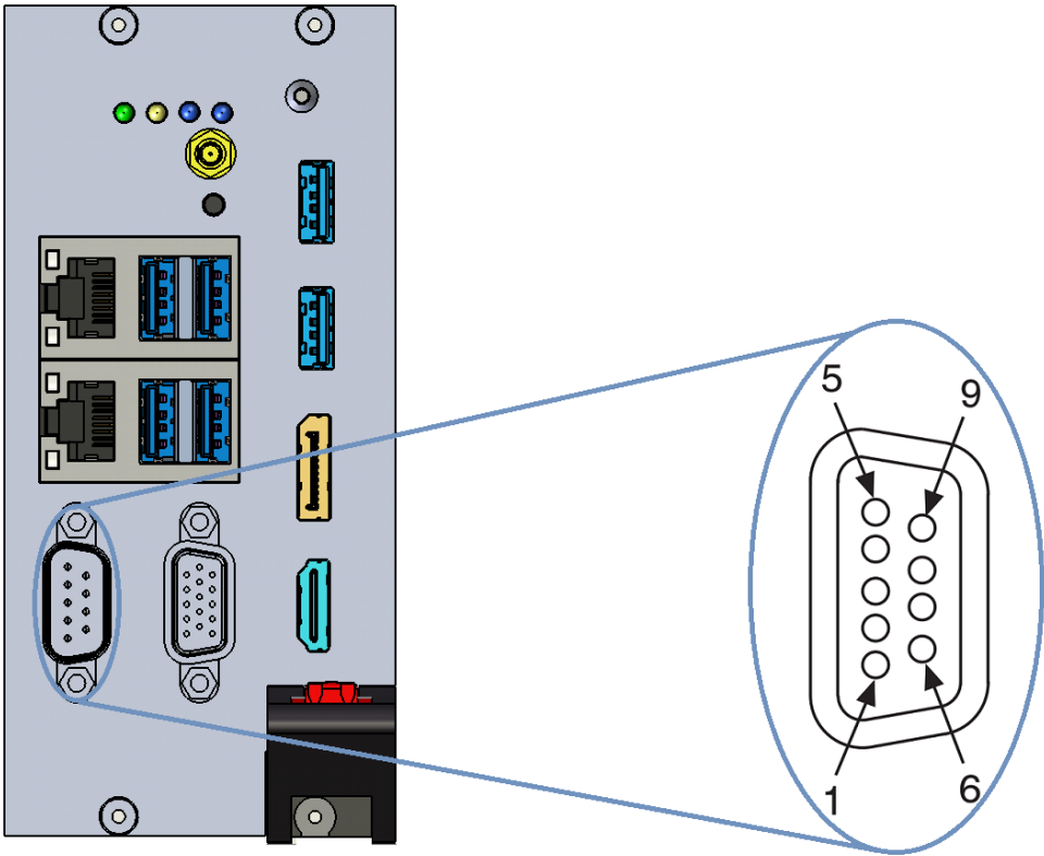
图 3-4 COM 接口示意图
