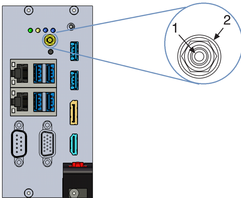
图 3-8 触发接口示意图
