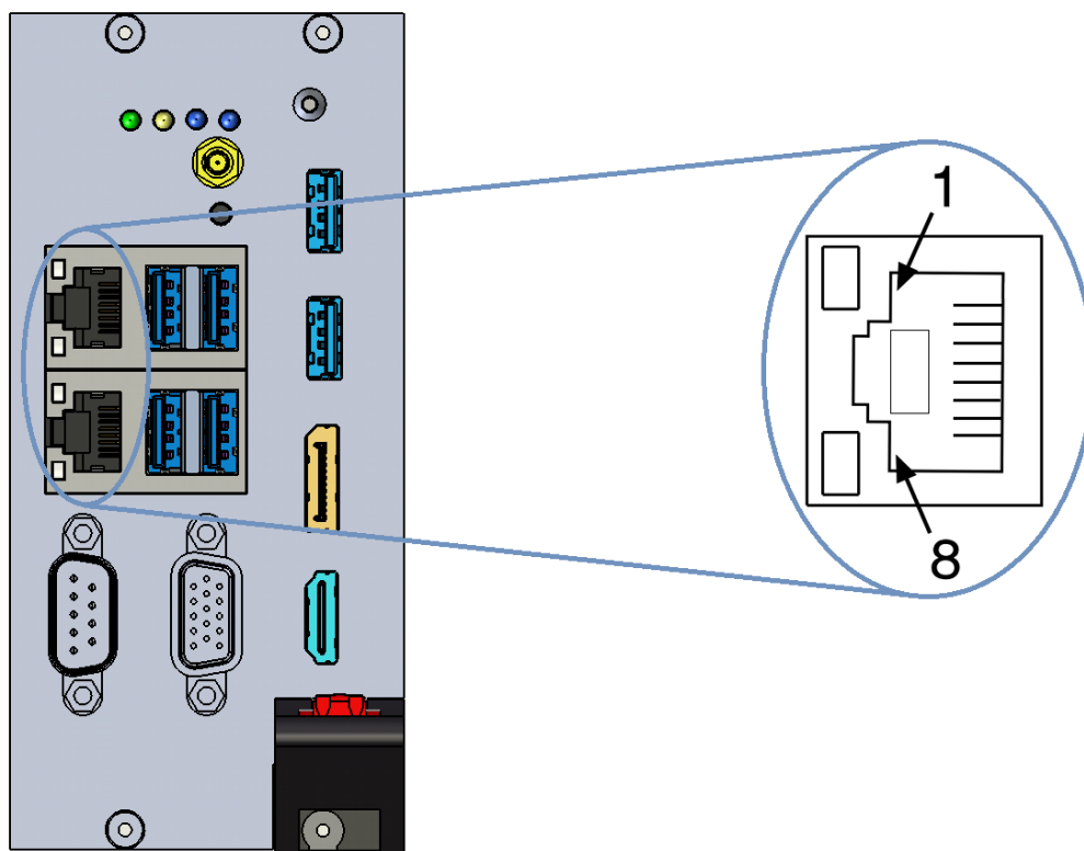
图 3-5 以太网接口示意图
