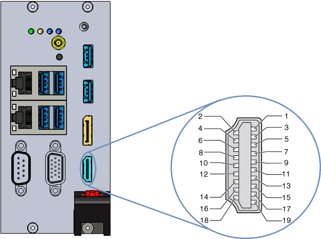
图 3-1 HDMI 接口示意图
