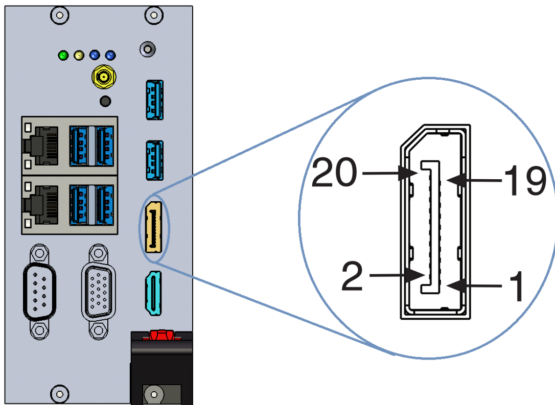
图 3-2 DP 接口示意图
