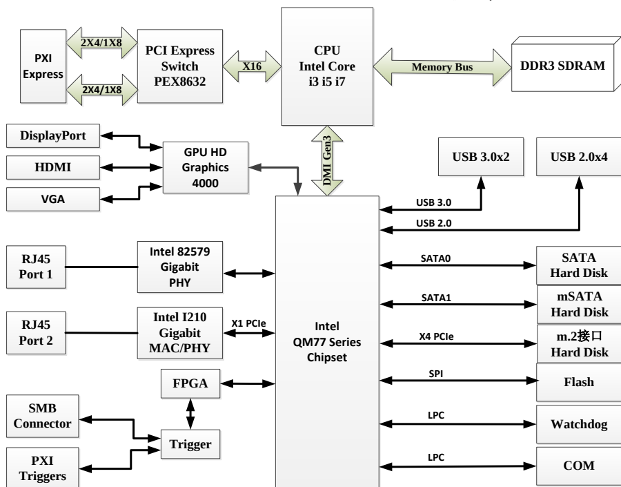
图 1-1 搭载 i7-3517UE CPU 系统功能框图
