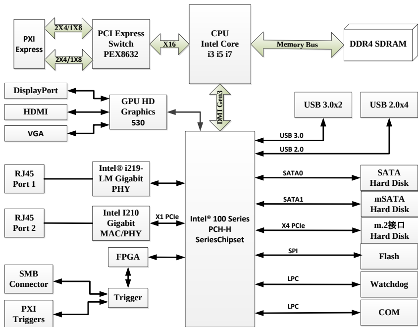
图 1-2 搭载 i7-6820EQ/6822EQ、i5-6440EQ、i3-6100E CPU 系统功能框图
