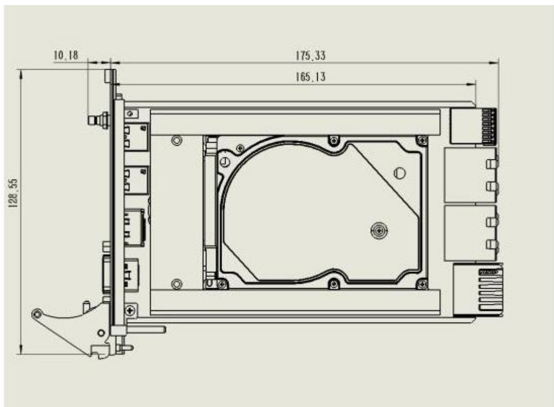
图 2-1 产品尺寸图
