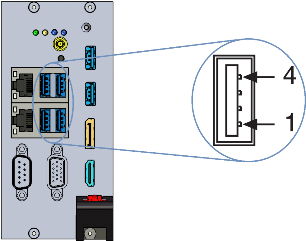
图 3-7 USB2.0 接口示意图
