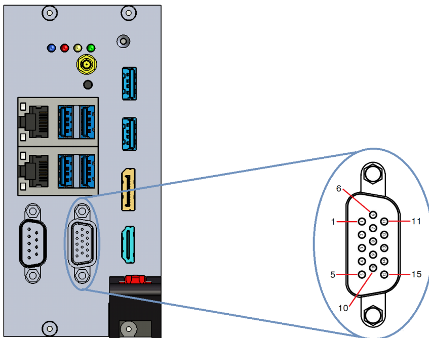
图 3.3 VGA 接口示意图
