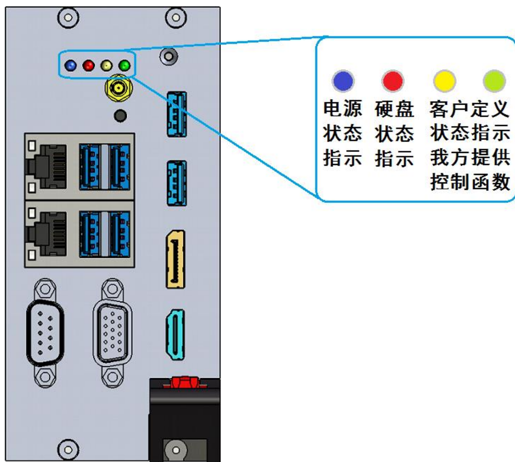
图 3-9 指示灯含义示意图
