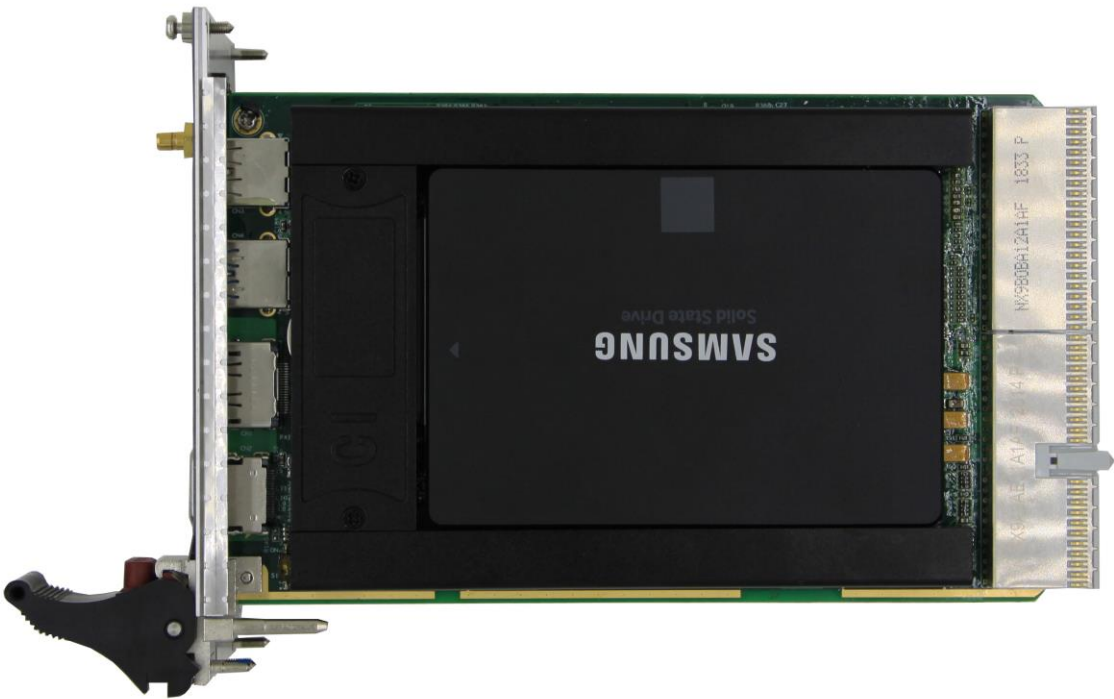
图 2-1 PXI-3873 产品侧视布局图
