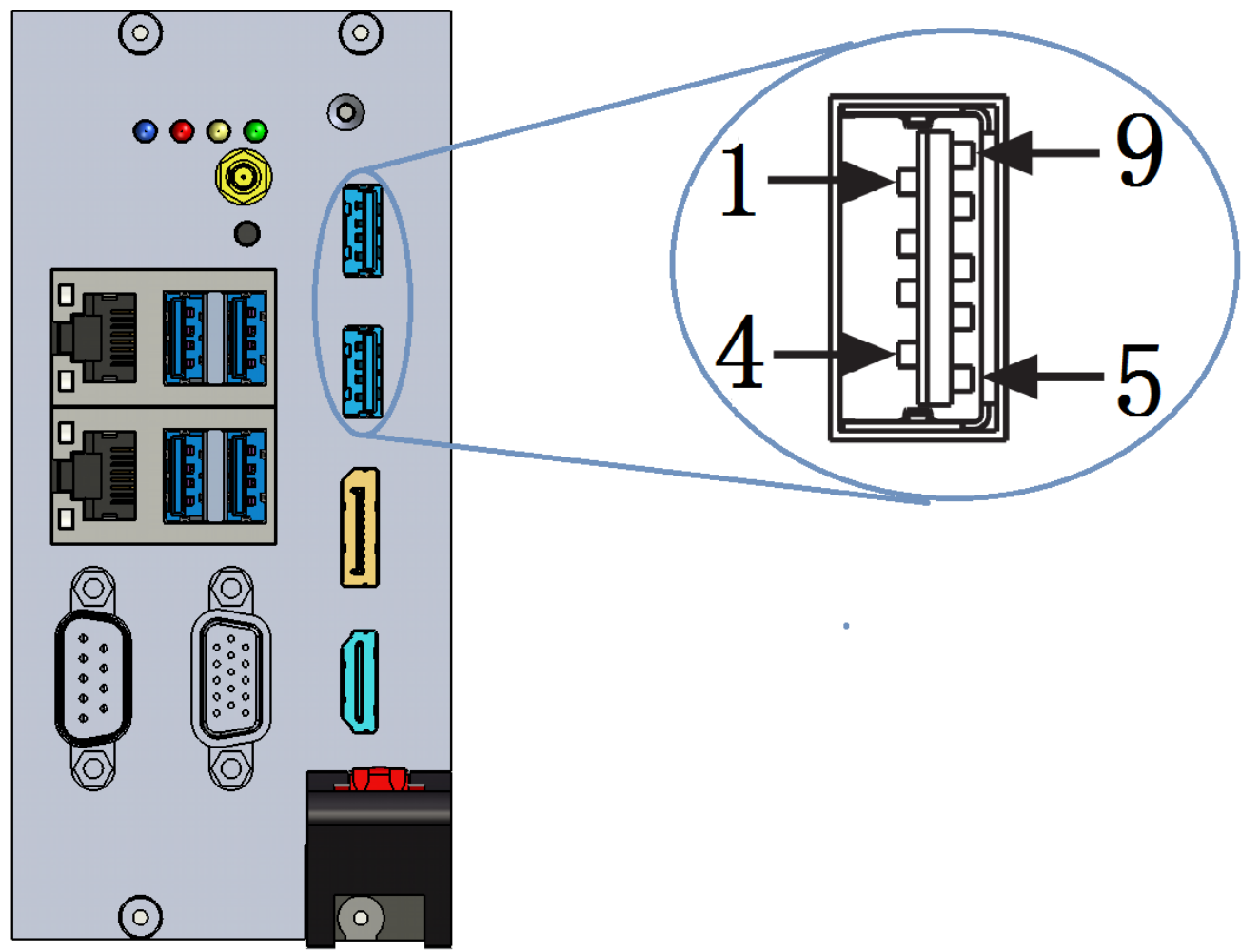
图 3-6 USB3.0 接口示意图
