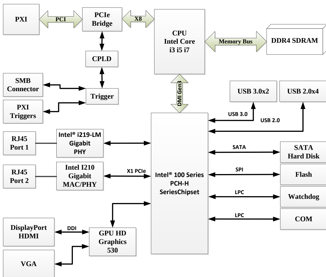
图 1-2 搭载 i7-6820EQ/6822EQ、i5-6440EQ、i3-6100E CPU 系统功能框图
