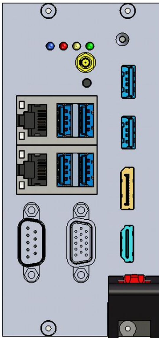
图 2-2 PXI-3873 产品面板布局图
