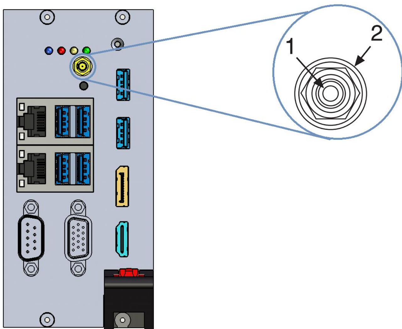
图 3-7 触发接口示意图
