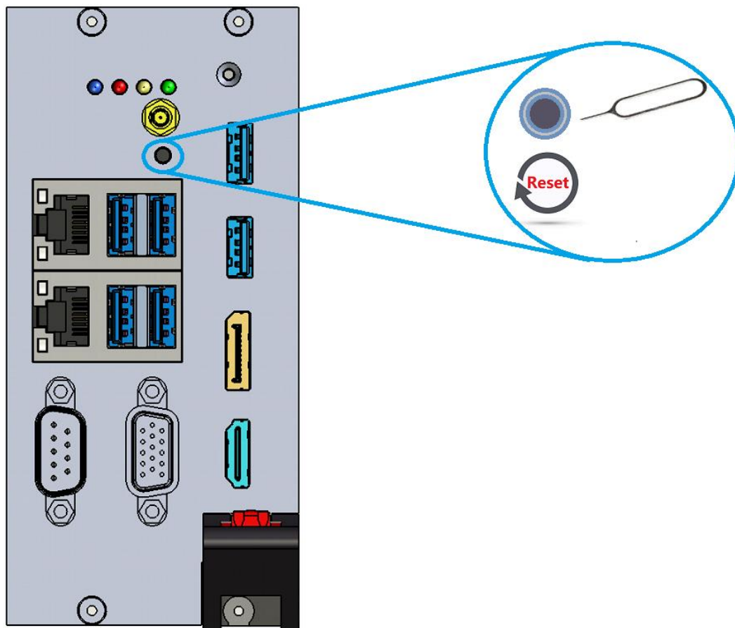
图 3-8 复位接口示意图
