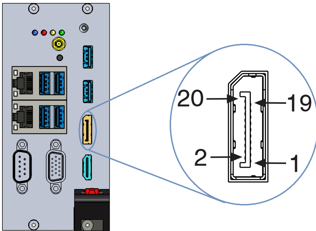
图 3-1 DP 接口示意图
