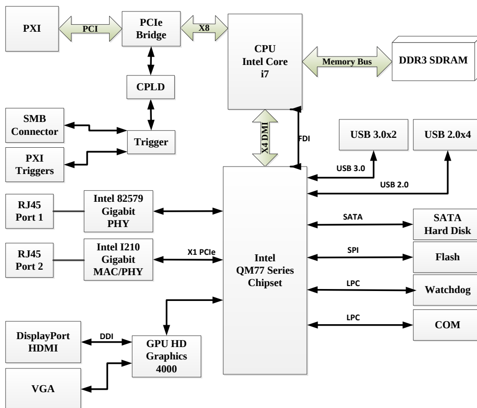
图 1-1 搭载 i7-3517UE CPU 系统功能框图
