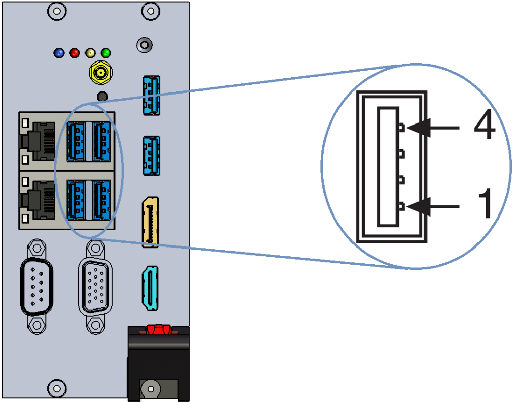
图 3-5 USB2.0 接口示意图
