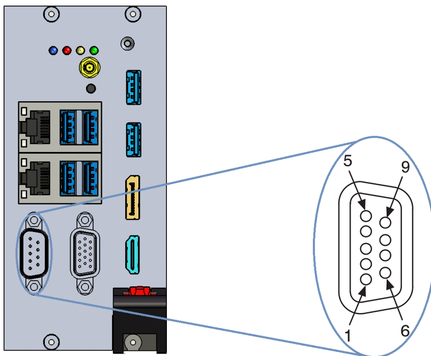
图 3-3 COM 接口示意图
