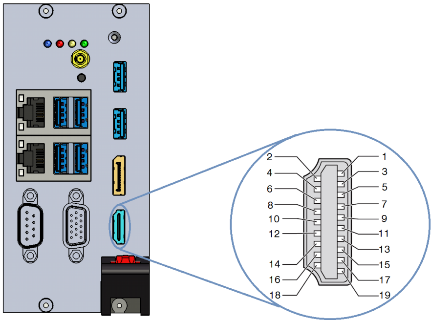
图 3-3 HDMI 接口示意图
