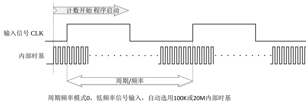
图 4-7 频率周期模式 0
