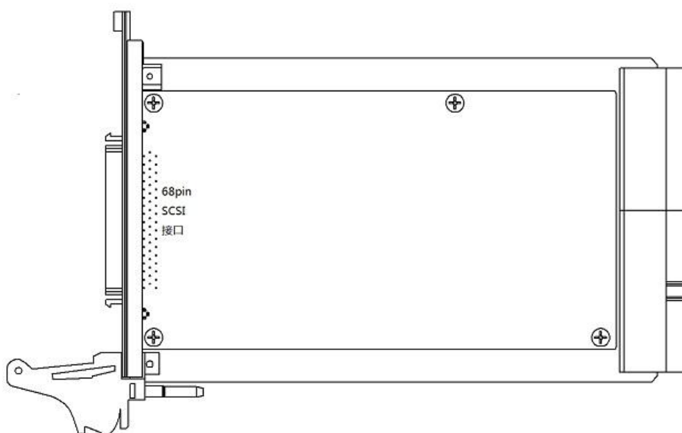
图 2-1 PXI-6261 产品布局图
