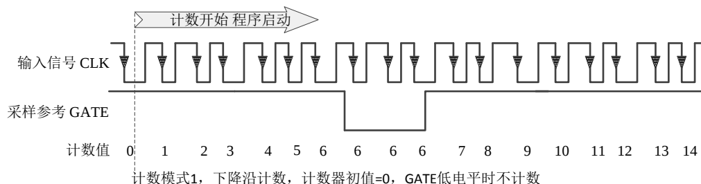
图 4-6 计数模式 1
