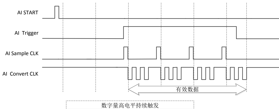
图 4-3 持续触发模式
