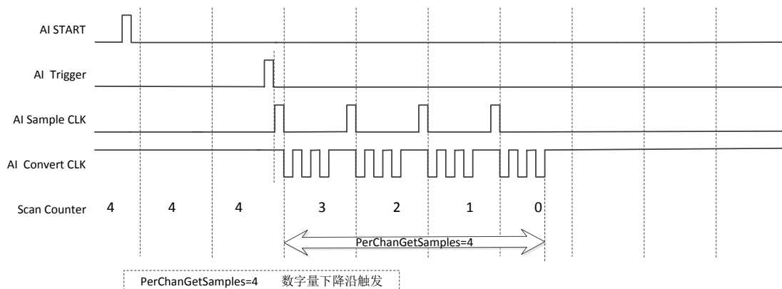
图 4-2 后触发模式
