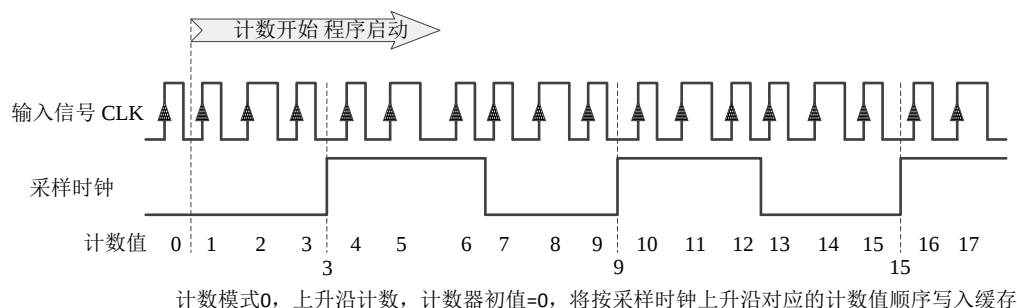
图 4-5 计数模式 0
