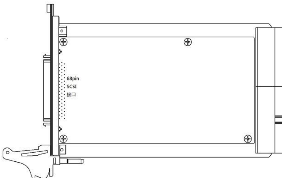
图 2-1 PXI-6772 产品布局图
