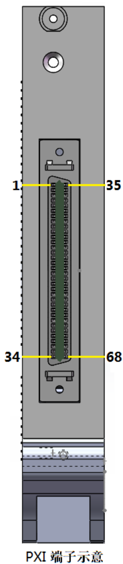
图 3-1 端子示意图
