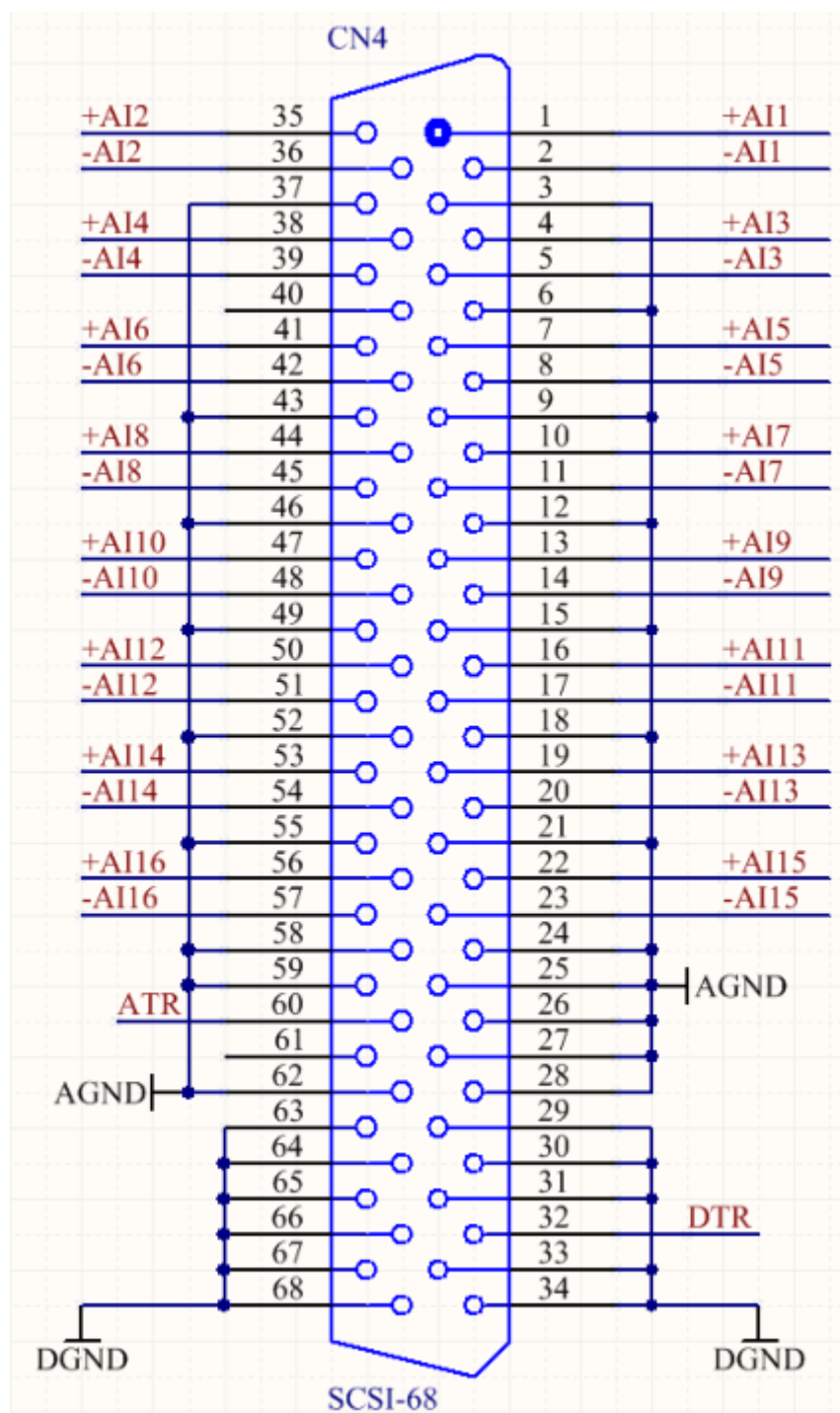
图 3-3 68-pin scsi 接口定义
