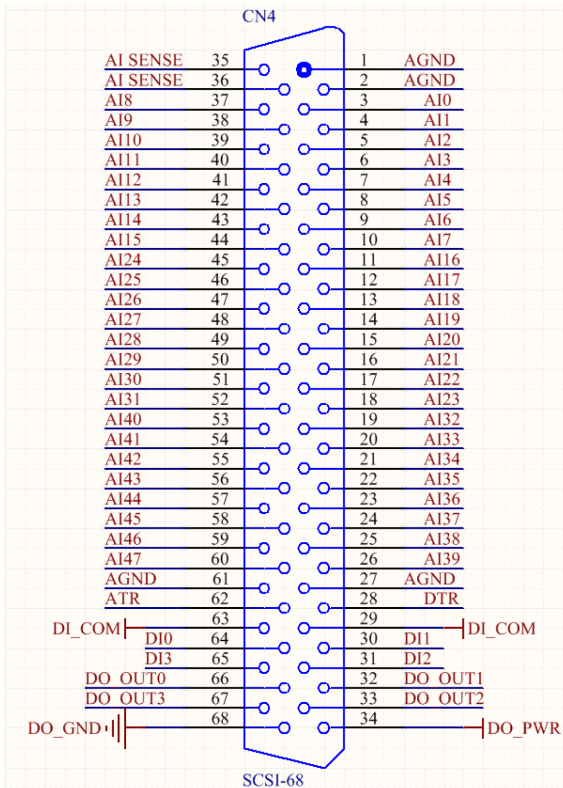
图 3-2 SCSI-68 端子原理图
