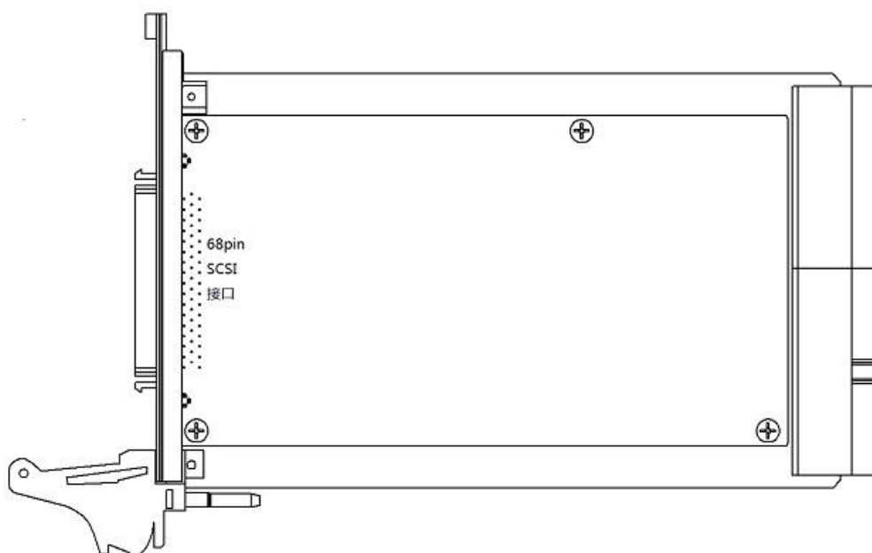
图 2-1 PXI-7265 产品布局图
