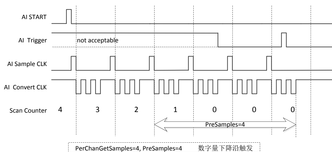
图 4-2 预触发模式
