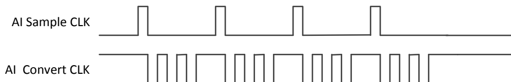
图 4-1 AI 工作时钟
