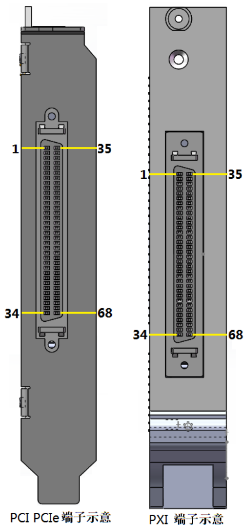
图 3-1 端子示意图
