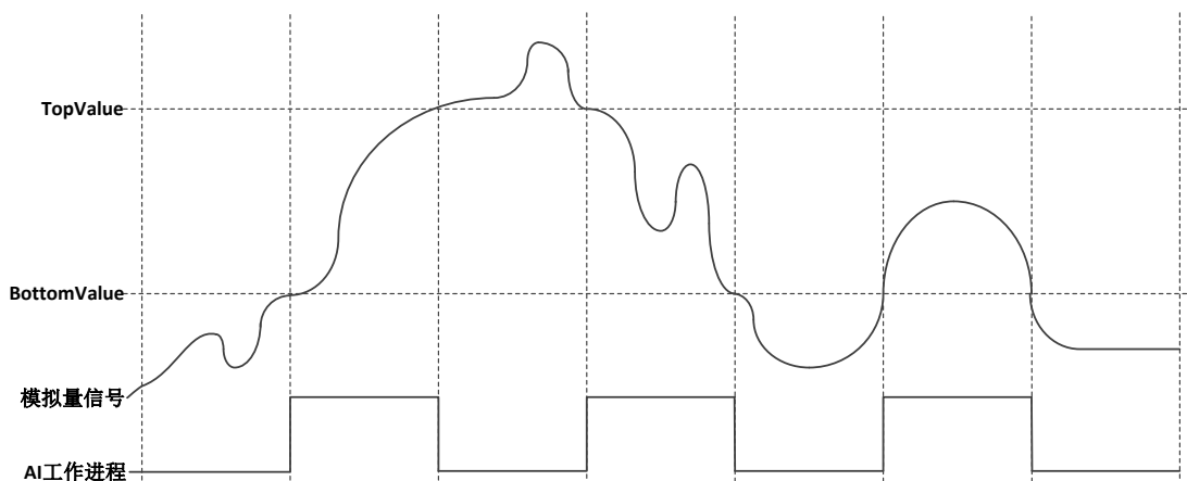
图 4-8 窗触发
